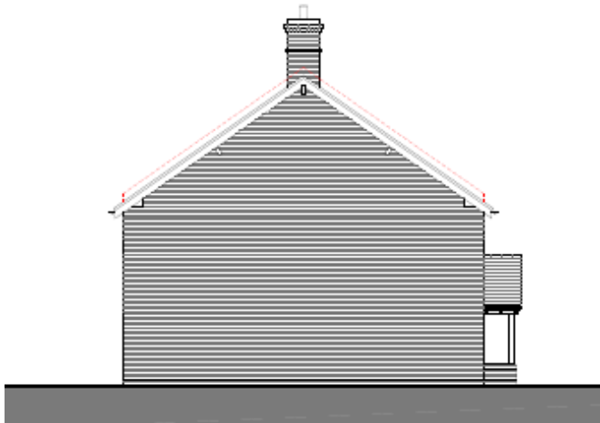
04 SIDE ELEVATION 1:50
