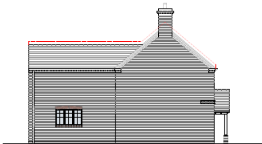
03 SIDE ELEVATION 1:50
