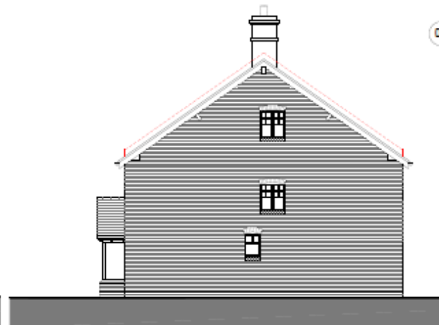
04 SIDE ELEVATION 1:50
